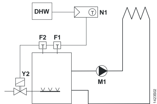
Прямое управление газовым напольным котлом и независимым управлением ГВС
