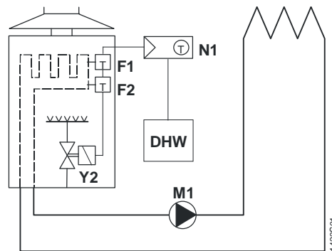
Прямое управление газовым настенным котлом и независимым управлением ГВС
