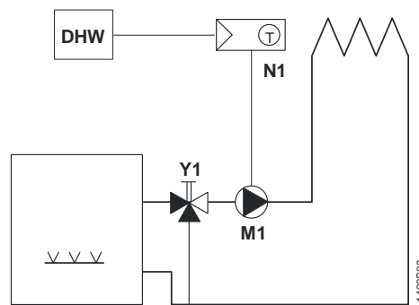
Прямое управление насосом контура отопления (предконтроль смешивающим клапаном вручную) и независимое управление ГВС
